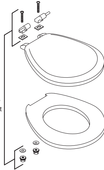
85057** Hinge Kit
