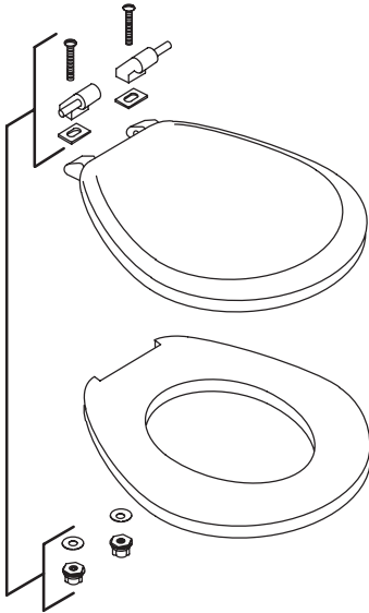
85057** Hinge Kit
