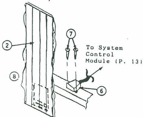
DOOR INTERLOCK DETAIL
