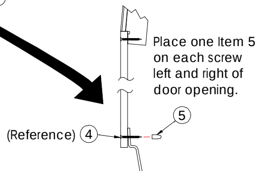
SKIRT DOOR DETAIL
